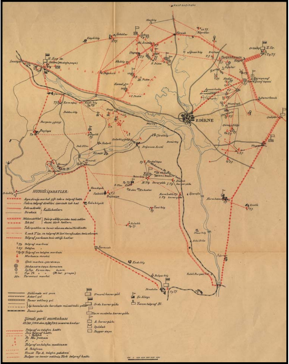
Ek-31: Kuşatma Ordusunun Muhabere Şebekesi
