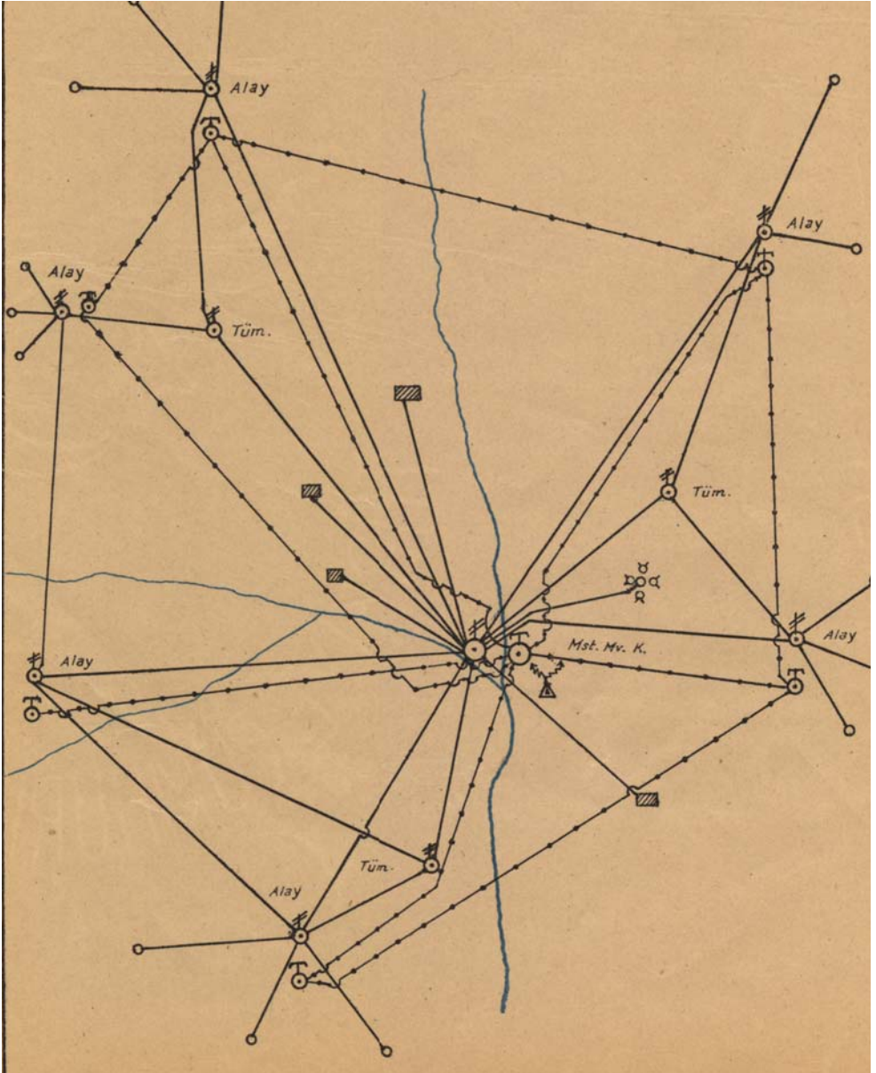
Ek-30: Edirne Kalesi'nin Muharebe Şebekesi (şema şeklinde)
