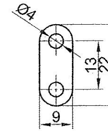
KALINLIK:0,5mm 2 NOLU PARÇA (KÖPRÜLEME PARÇASI)
