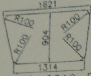
6250-0019-P
