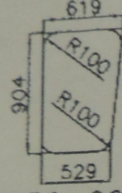
6250-0021-P
