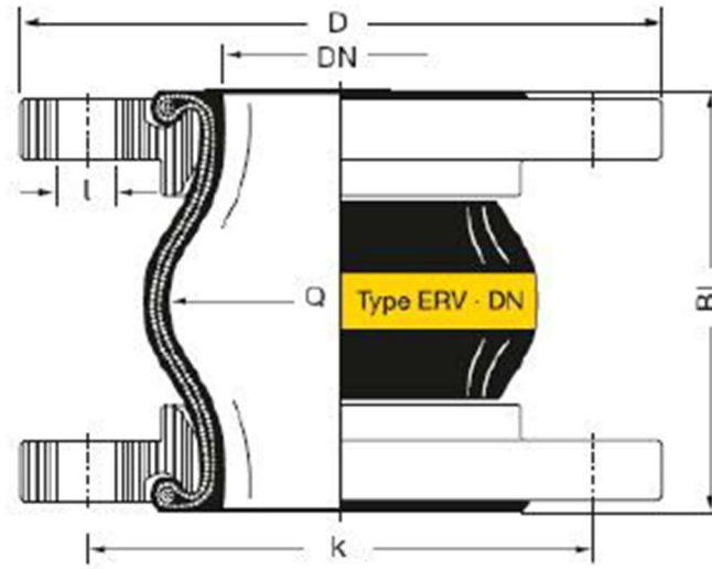
Şekil 1.21 Kompansatör, Lastik, DN50
