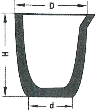
Şekil: Grafit pota şekli ve ölçüleri (toleranslı aralıklar aşağıda verilmiştir).
