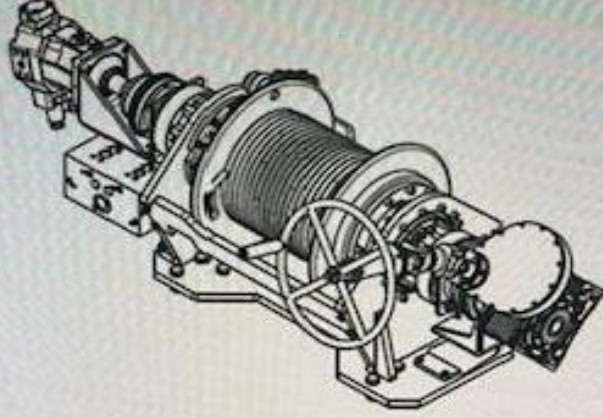
Şekil 1.3 Baş Kapak İrgat Komple
