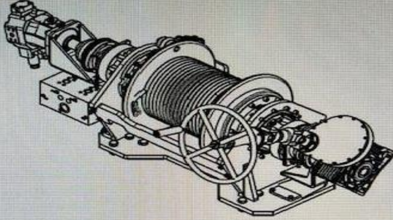
Şekil 1.4 Baş Kapak Tambur Sistemi
