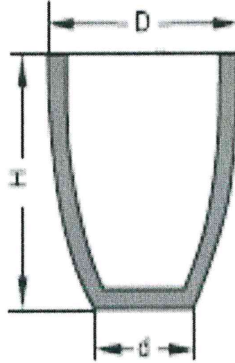
Şekil: Grafit pota şekli ve ölçüleri (toleranslı aralıklar aşağıda verilmiştir).
