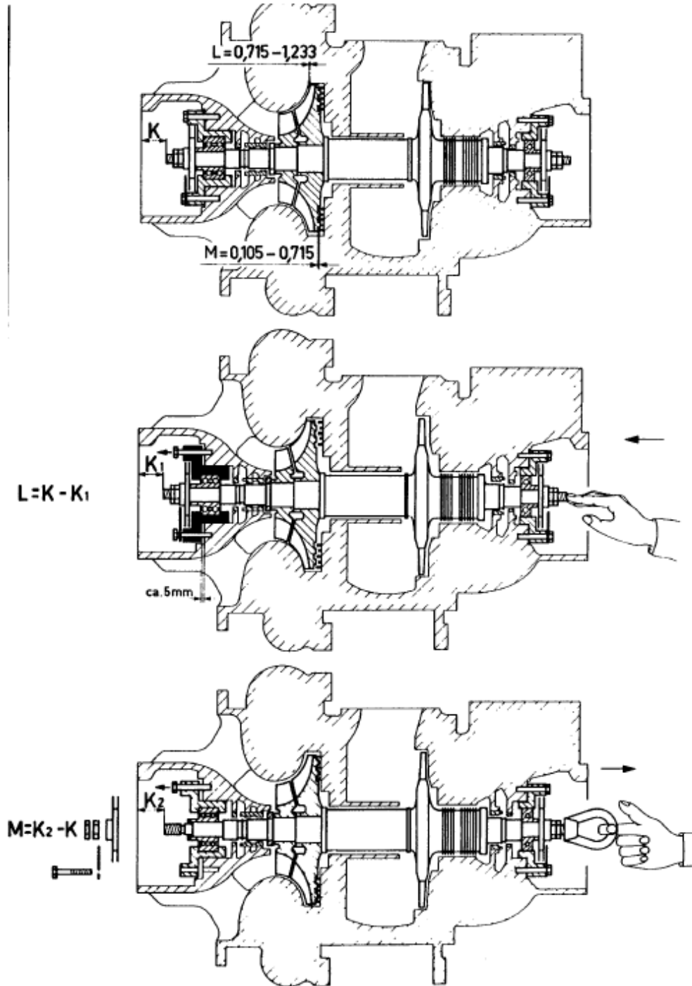
Şekil.2 MTU 16V 652 Turboşarjerine ait ölçüler
