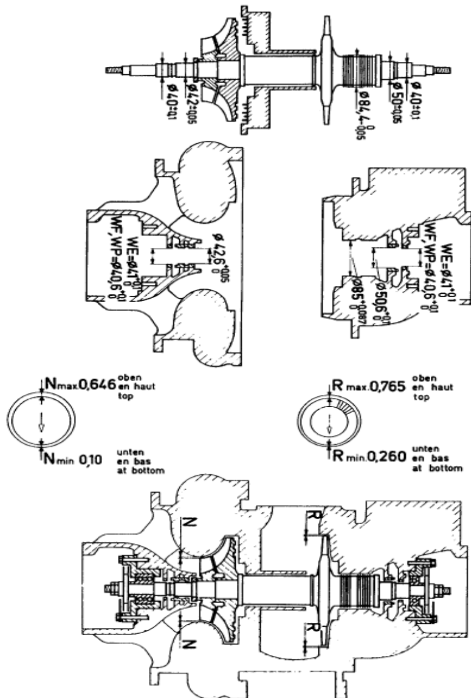
Şekil.1 MTU 16V 652 Turboşarjerine ait ölçüler
